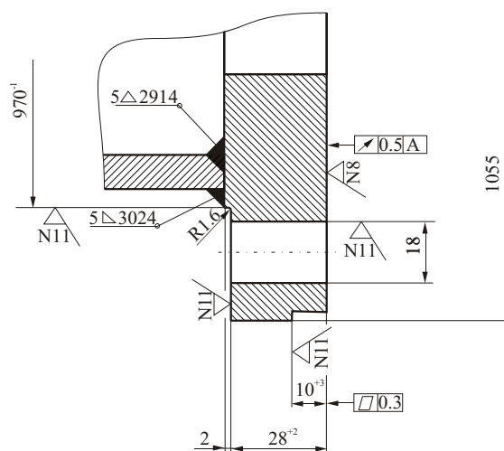
DETALJ "Z" M 1:2
