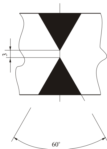
Detalj "X"
