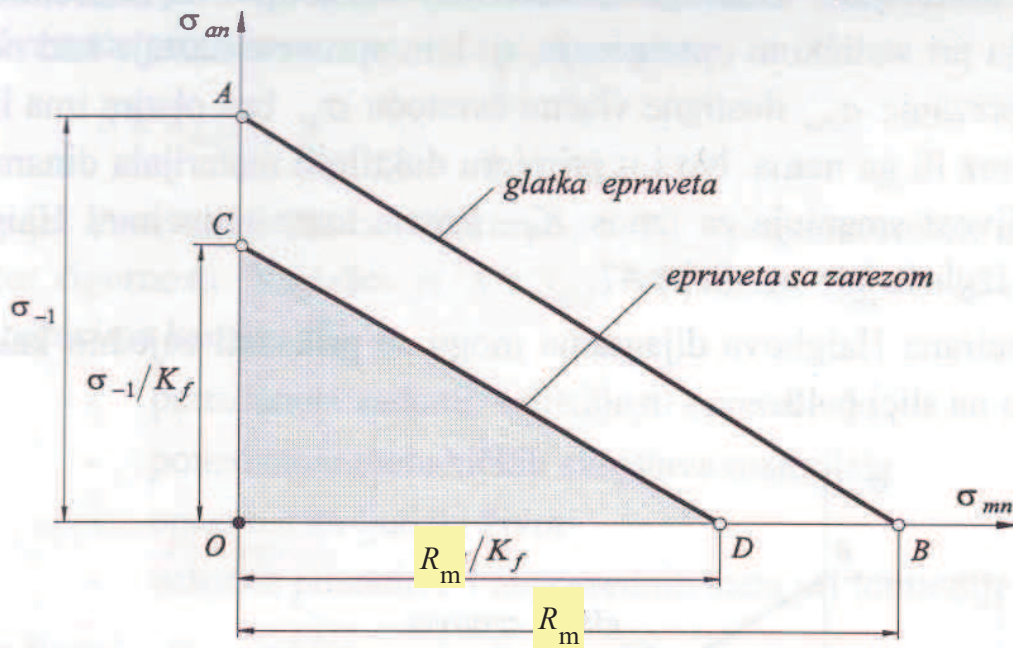
Slika 6.46 Reducirani Haighov dijagram za epruvetu od krhkog materijala sa zarezom
