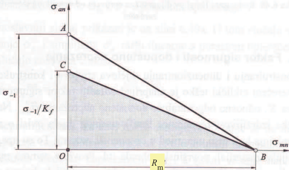
Slika 6.47 Reducirani Haighov dijagram za epruvetu od duktilnog materijala sa zarezom
