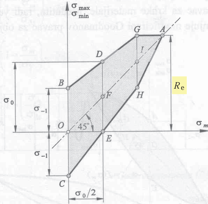
Slika 6.37 Smithov dijagram shematiziran pomoću \sigma_{-1} i \sigma_0
