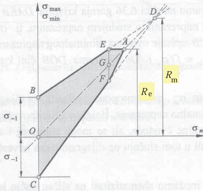
Slika 6.38 Jednostavnija shematizacija Smithova dijagrama
