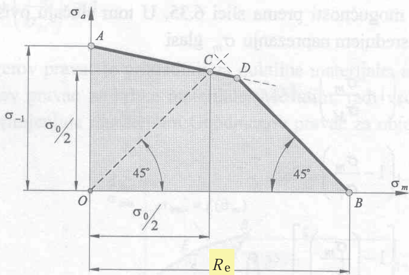
Slika 6.33 Shematizirani Haighov dijagram prema Serensenu i Kinosošviliju
