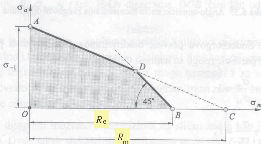
Slika 6.34 Jednostavnija shematizacija Haighova dijagrama
