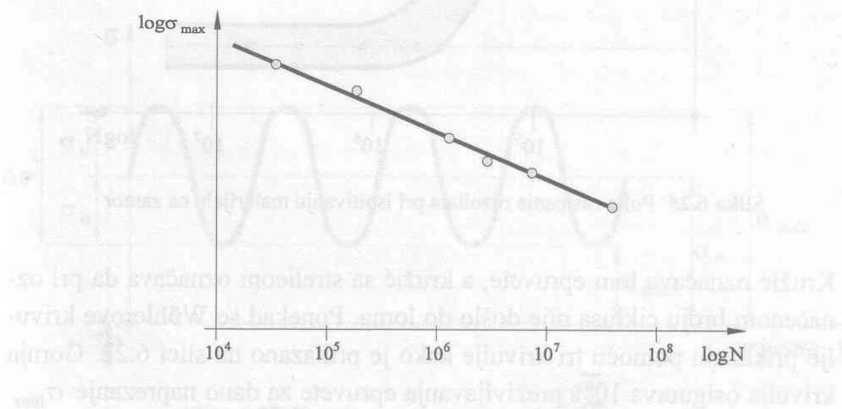
Slika 6.24 Wöhlerova krivulja u logaritamskom mjerilu
