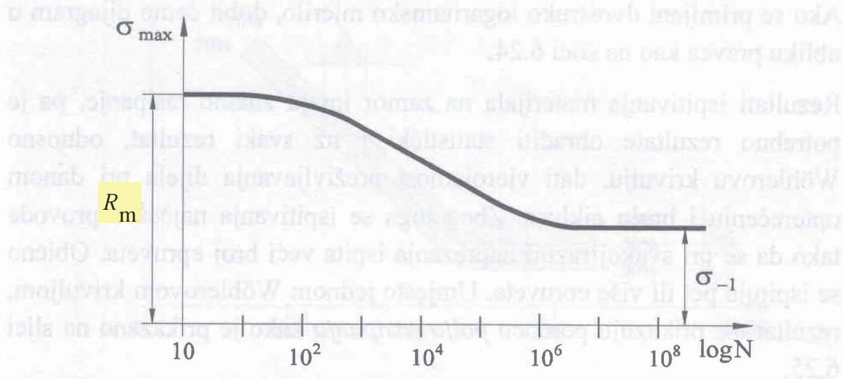
Slika 6.23 Wöhlerova krivulja u polulogaritamskom mjerilu
