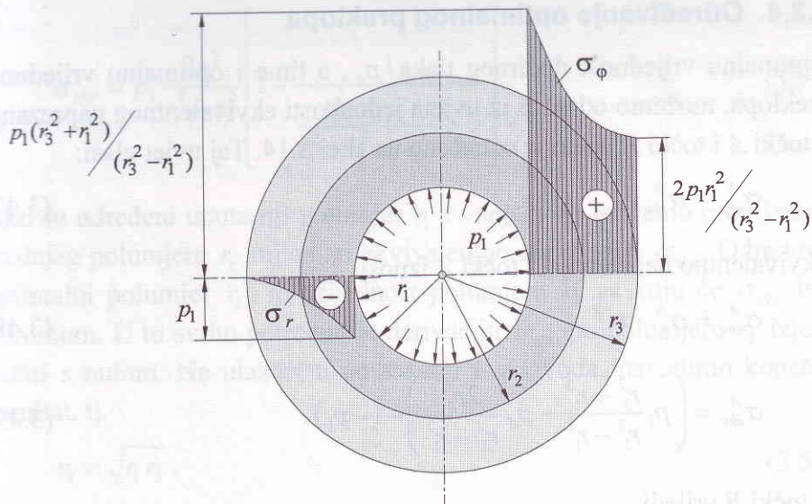
Slika 3.13 Raspodjela naprezanja u sastavljenoj cijevi koja nastaju pod djelovanjem unutarnjeg tlaka p_1
