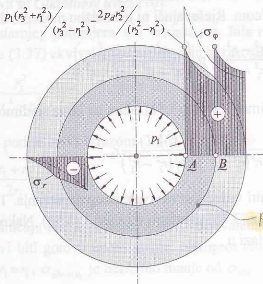
Slika 3.14 Raspodjela naprezanja u sastavljenoj cijevi koja nastaju pod djelovanjem dodirnog tlaka p_d i unutarnjeg tlaka p_1
